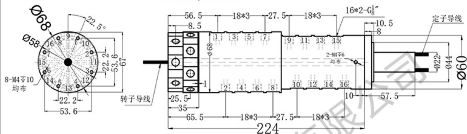
气滑环参数
